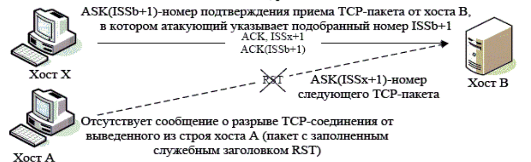
Рисунок 7. Схема реализации угрозы "Подмена доверенного объекта сети"
