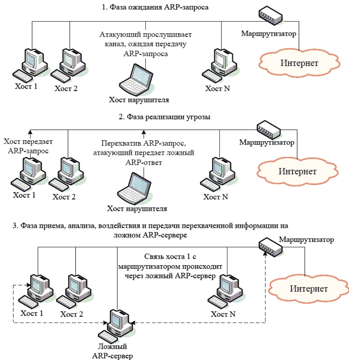
Рисунок 10. Схема реализации угрозы "Внедрение ложного ARP-сервера"
