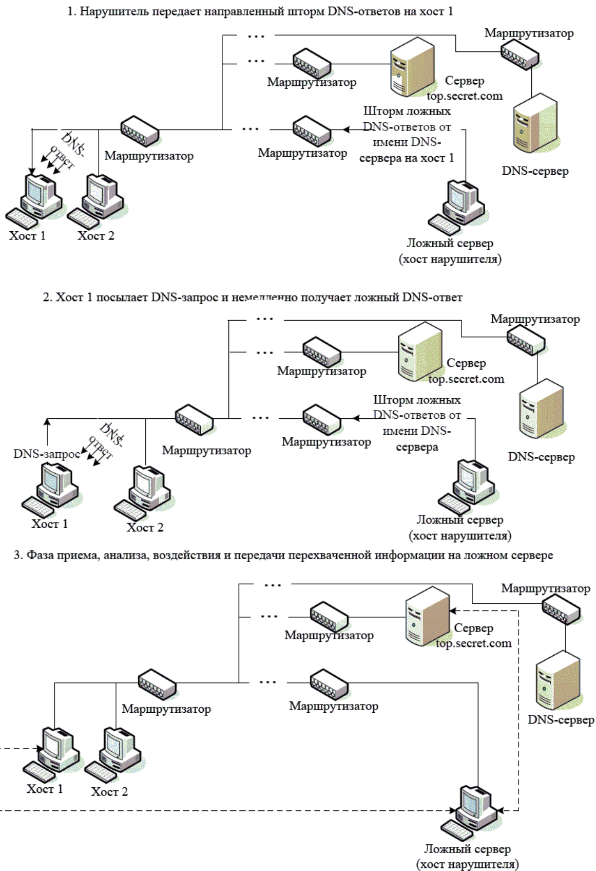
Рисунок 12. Схема реализации угрозы "внедрение ложного DNS-сервера" путем шторма DNS-ответов на компьютер сети
