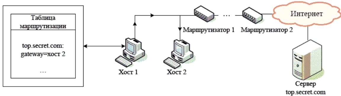
Рисунок 8. Схема реализации атаки "Навязывание ложного маршрута" (внутрисегментное) с использованием протокола ICMP с целью нарушения связи
