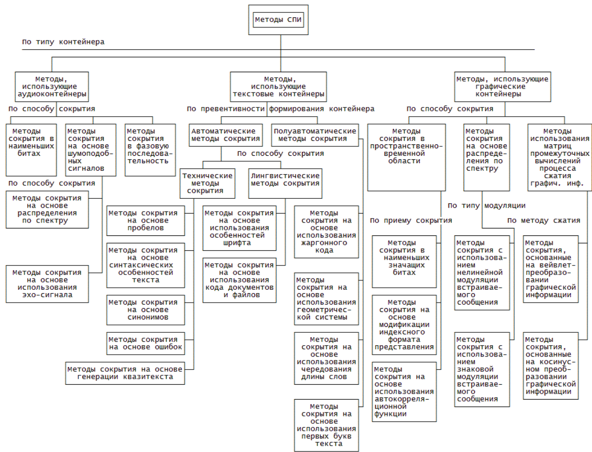
Рисунок 15. Классификация методов стеганографического преобразования информации (СПИ)
