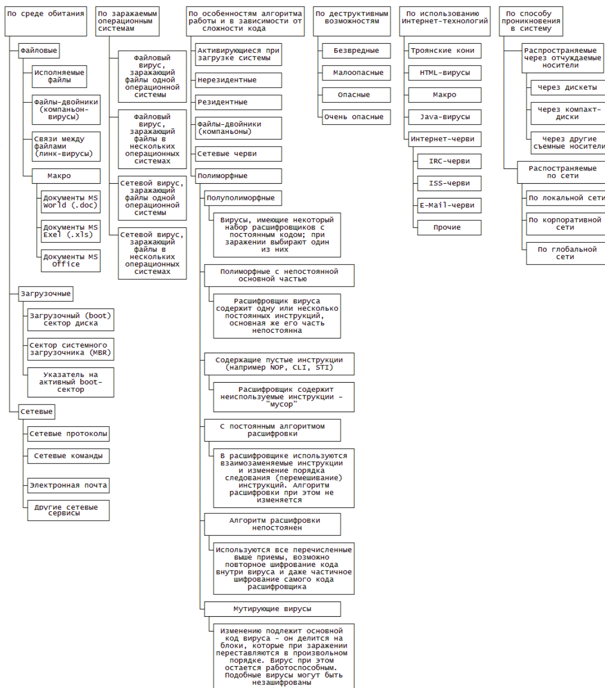
Рисунок 14. Классификация программных вирусов и сетевых червей
